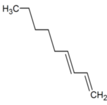
Nona-1,3-diene
